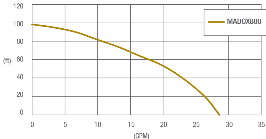
Curva de operación de la bomba
