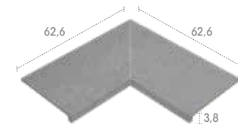
E62 62,6 x 62,6 x 3,8
