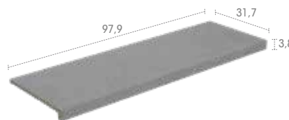
L98 97,9 x 31,7 x 3,8
